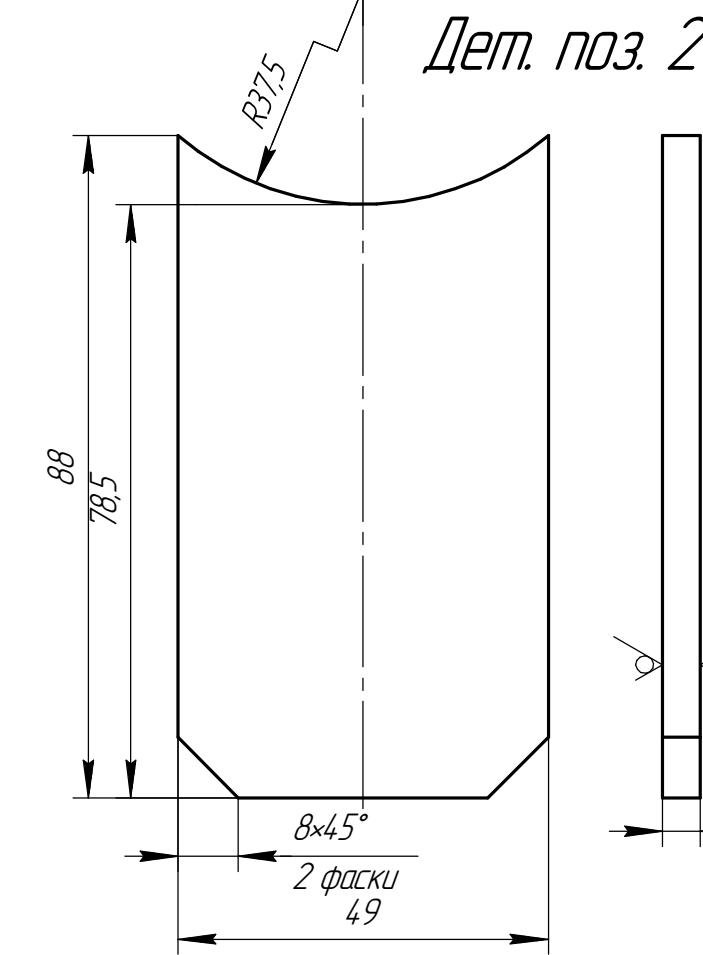
Дет. поз. 2 (2:1)
