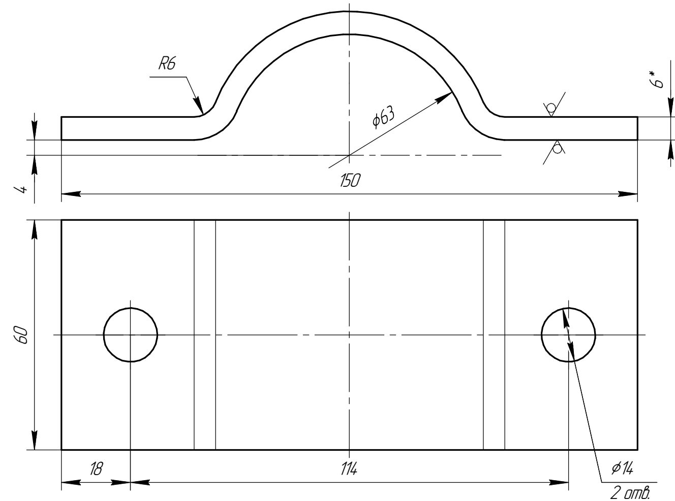
Дет. поз. 6 (1:2)
