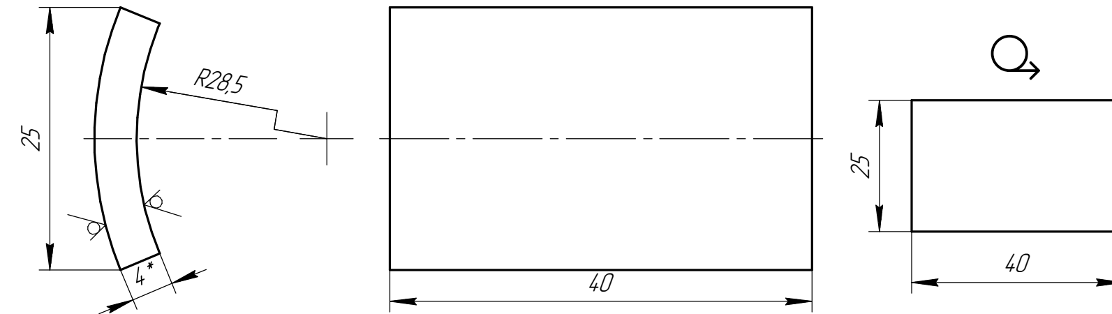
Дет. поз. 2 (2:1)
