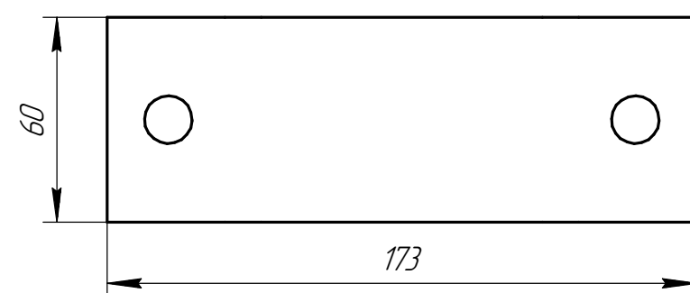
Дет. поз. 6 (1:2)
